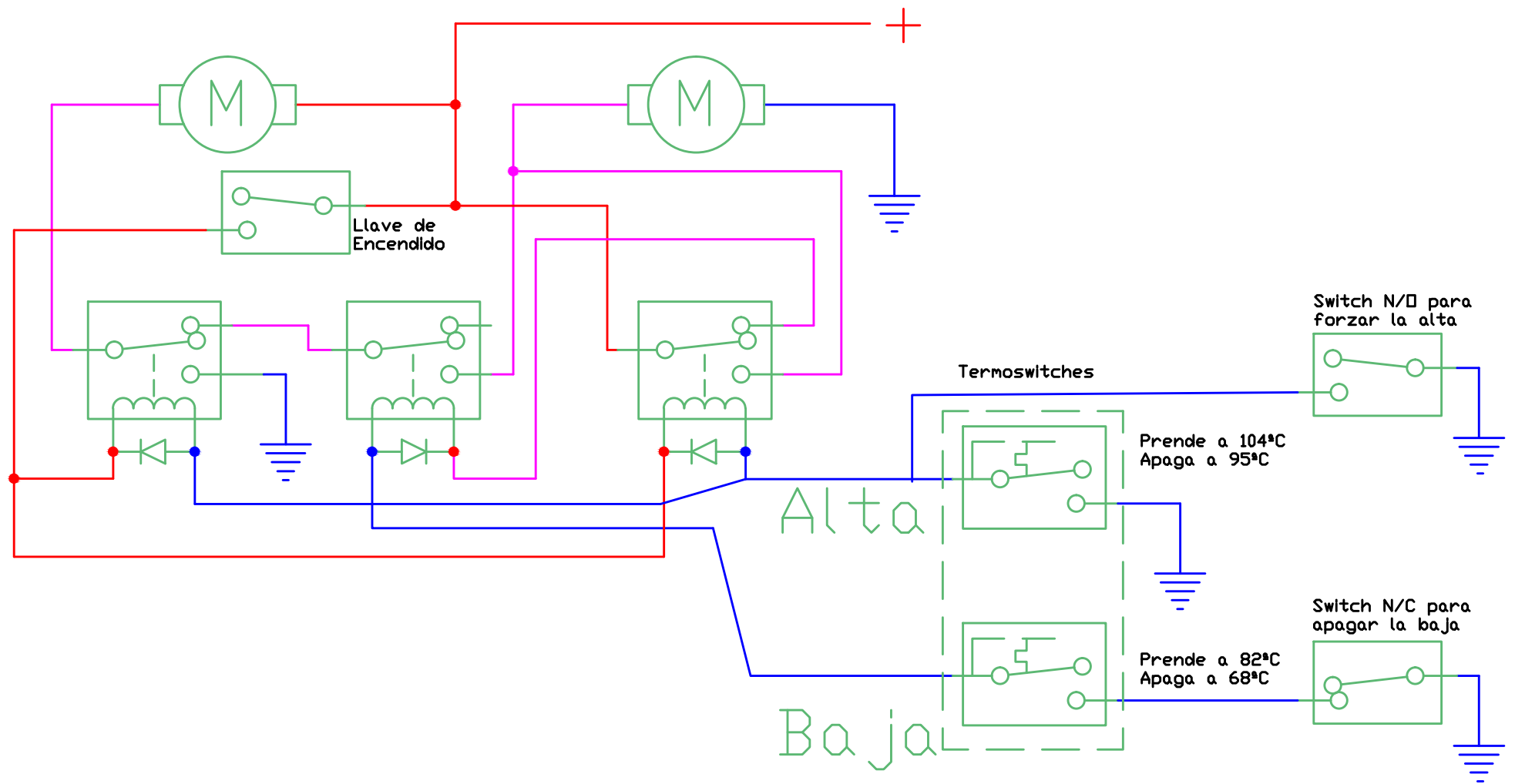
Circuito de Dos Velocidades para Dos Ventiladores.
